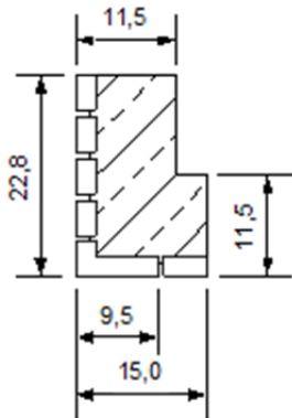
normale Bewehrung
